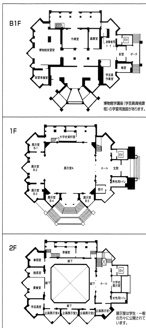
館内図面
